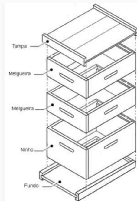
Figura 1 — Esquema de uma colmeia Langstroth completa
