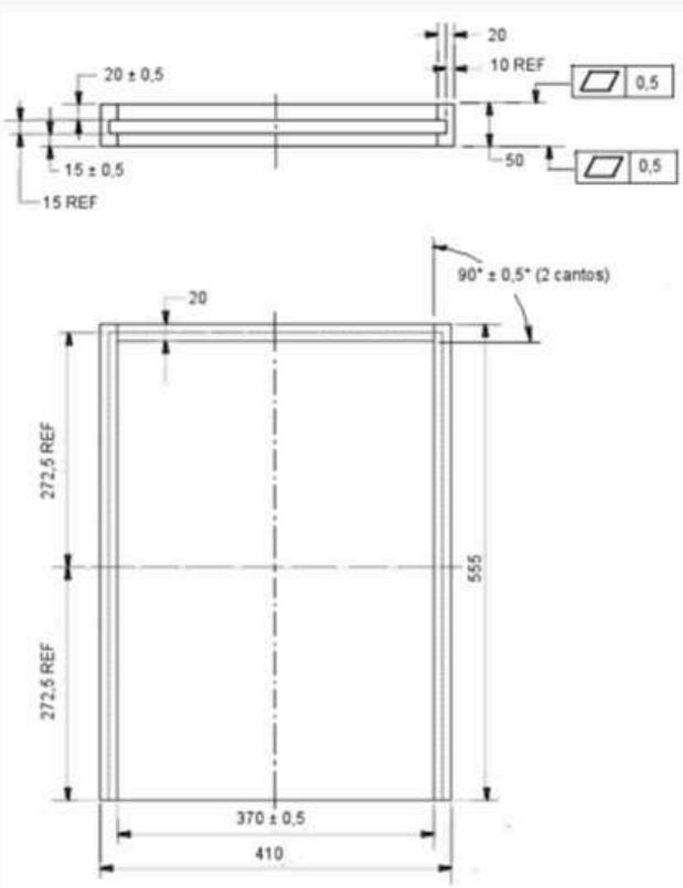
Figura 2 — Dimensões e tolerâncias do fundo montado
